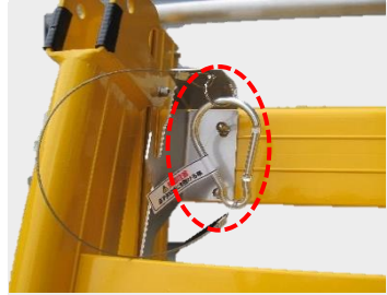
【④矢印板飛散防止フック】
